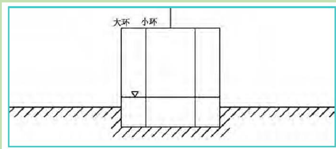
图 4.2-6 渗水试验装置示意图
