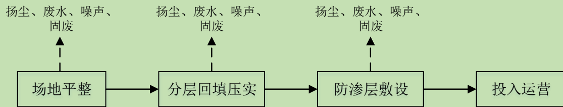
图 2.2-1 贮灰场施工工艺流程及产污环节图
