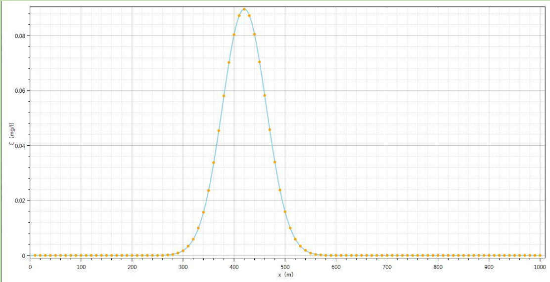
图 4.2-11 污染物在潜水层运移 3000d 时运移图
