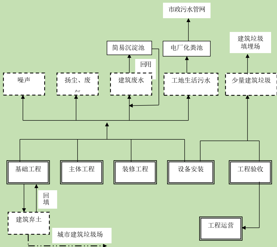
图 2.2-3 洗车间施工工艺流程及产污环节图
