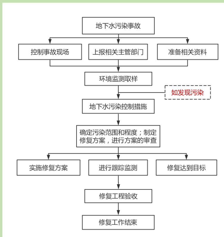
图 6.2-3 地下水污染应急治理程序框图
