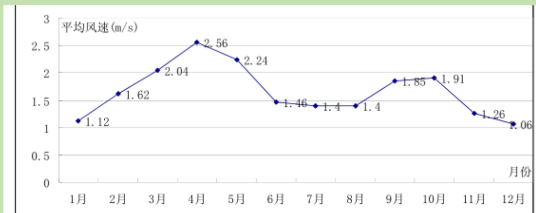
图4.2-2 年平均风速的月变化曲线图
