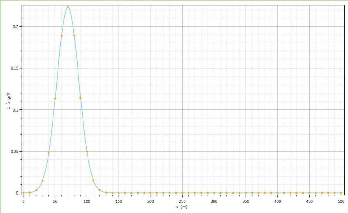
图 4.2-9 污染物在潜水层运移 500d 时运移图
