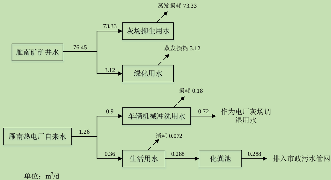
图 2.2-6 运营期水平衡图
