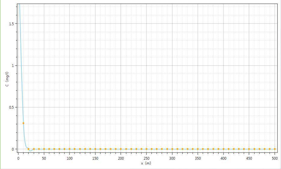
图 4.2-7 污染物在潜水层运移 30d 时运移图
